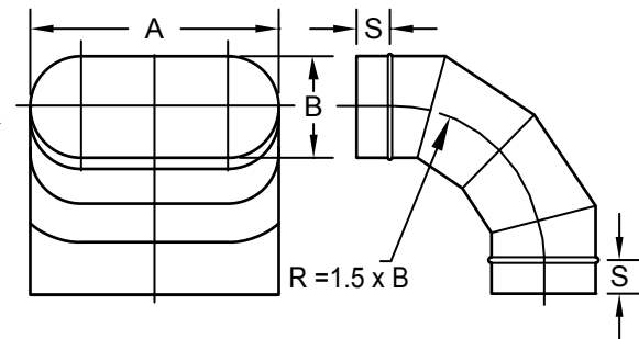
90° ANGLE EASY
